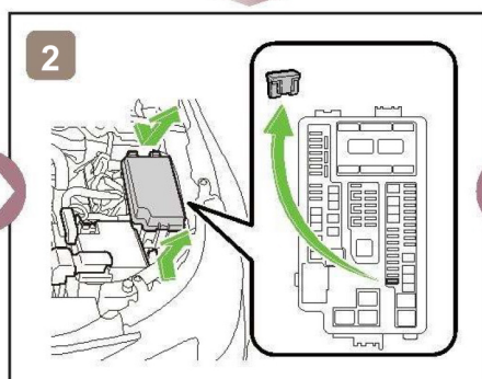
Fusível IG2-PRINCIPAL, 20 A AMARELO
